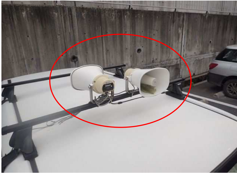
広報用スピーカー及びアンプ設置状況（参考）
