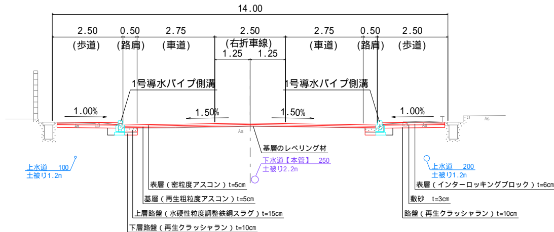
標準断面図
