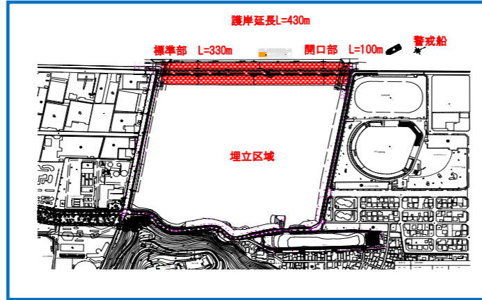
【標準施工図】
