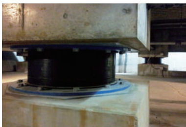
建物地下に設置された免震装置
