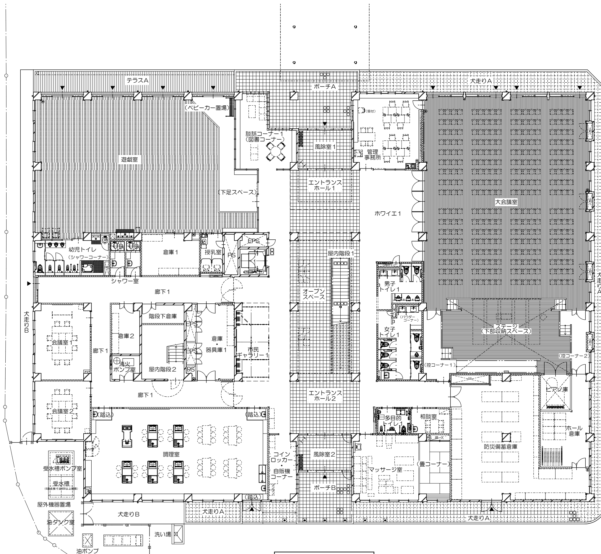
1階平面図
