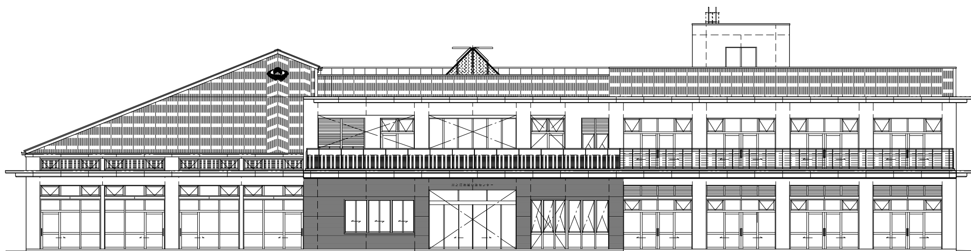
西面立面图
